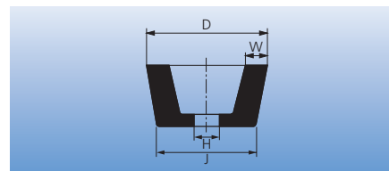
Коническая шлиф. чашка
